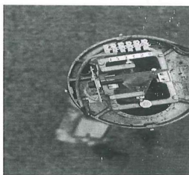
Limpieza del pluviómetro
