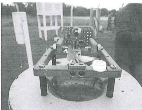
Mantenimiento preventivo del pluviómetro
