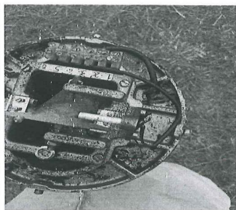
Mantenimiento preventivo del pluviómetro
